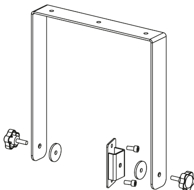
LDEB122G2SB / LDEB152G2SB Schwenkbügel
